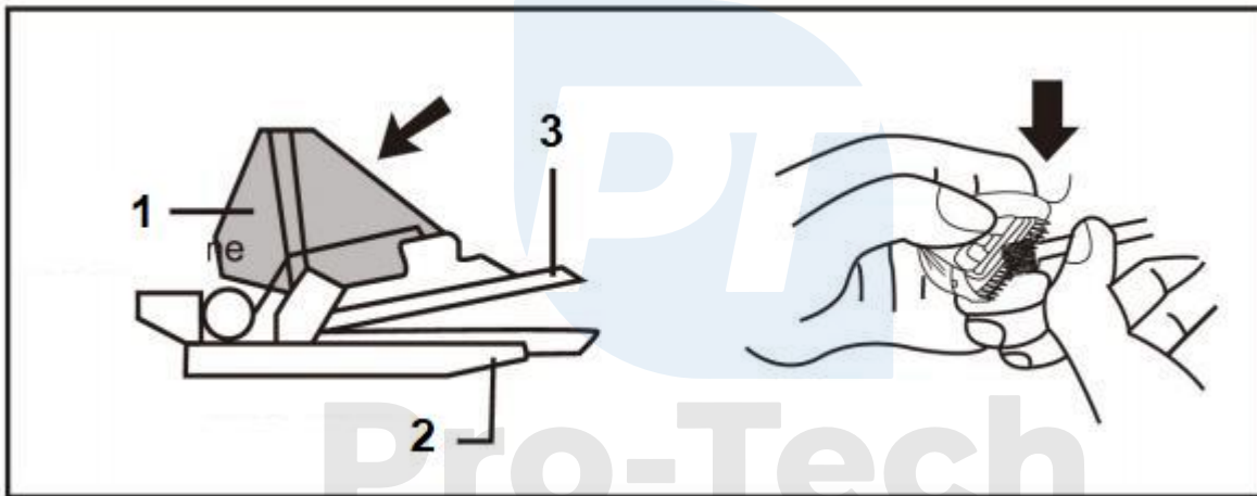
1. Rám s pohyblivou čepeľou 2. Statická čepeľ 3. Pohyblivá čepeľ
